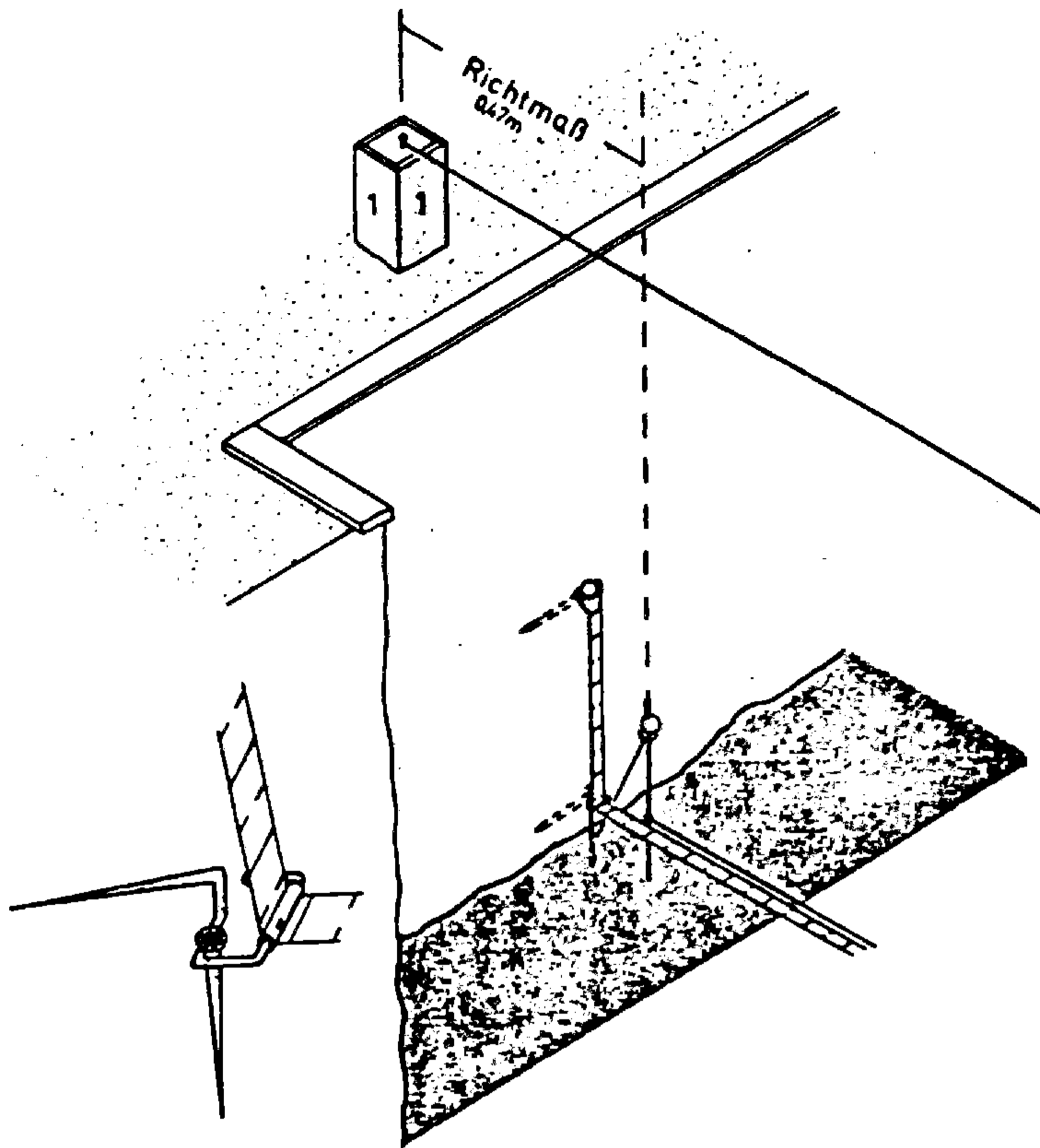
(شكل ١٦) طريقة رفع الموقع
